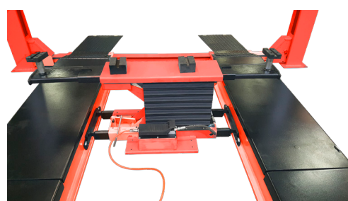
Elevador entre vías con bomba oleoneumática Lift sliding crosspieces with oleopneumatic pump
